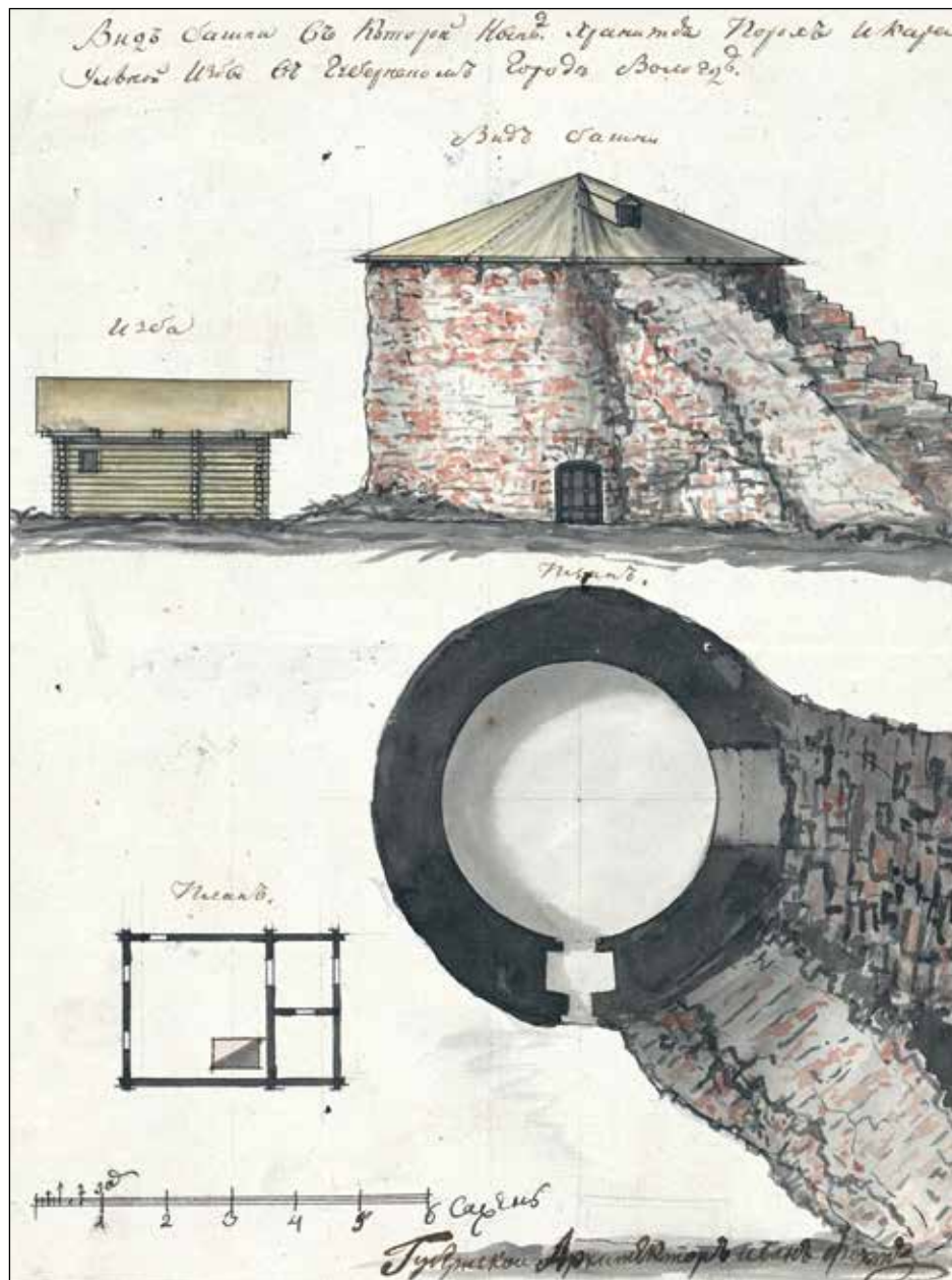
Чертеж Пречистенской (Пороховой) башни. Архитектор И. А. Фохт, 1809 г. Российский государственный исторический архив. Ф. 1488. Оп. 1. Д. 577. Л. 1
